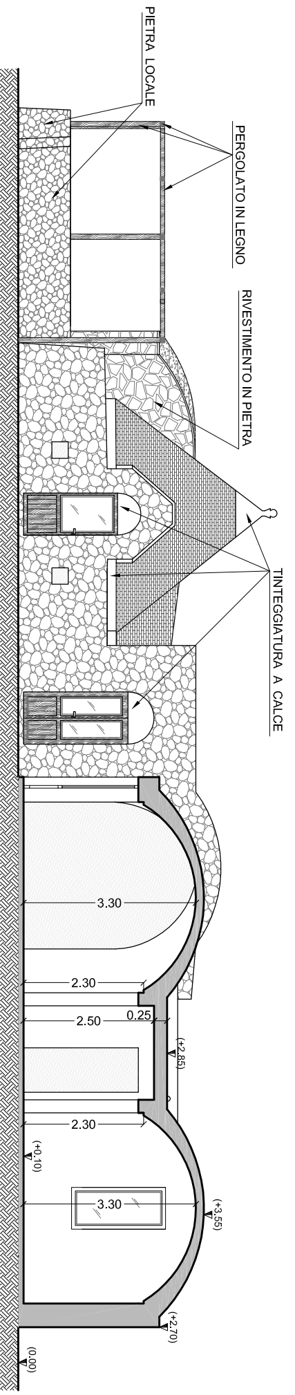
SEZIONE E - F DI PROGETTO
