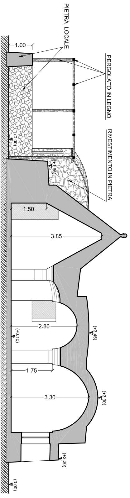
SEZIONE A - B DI PROGETTO
